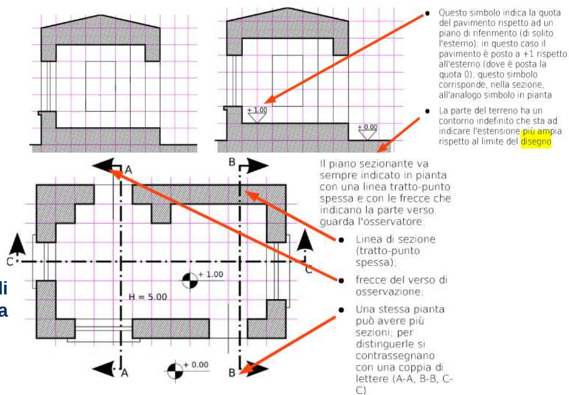
La sezione C-C:
