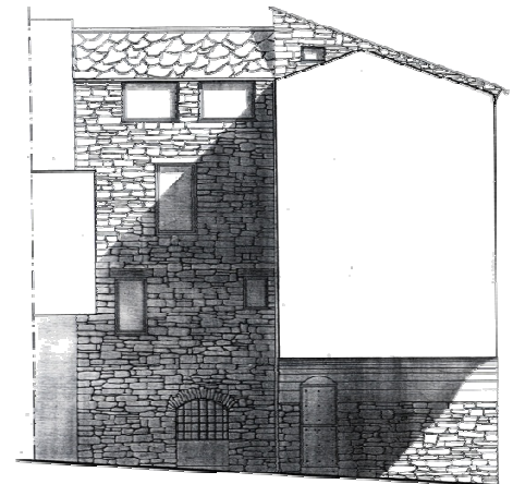
Prospetto Ovest Prospetto laterale Prospetto su Via Rossi
