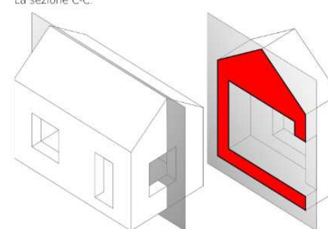
La sezione C-C:
